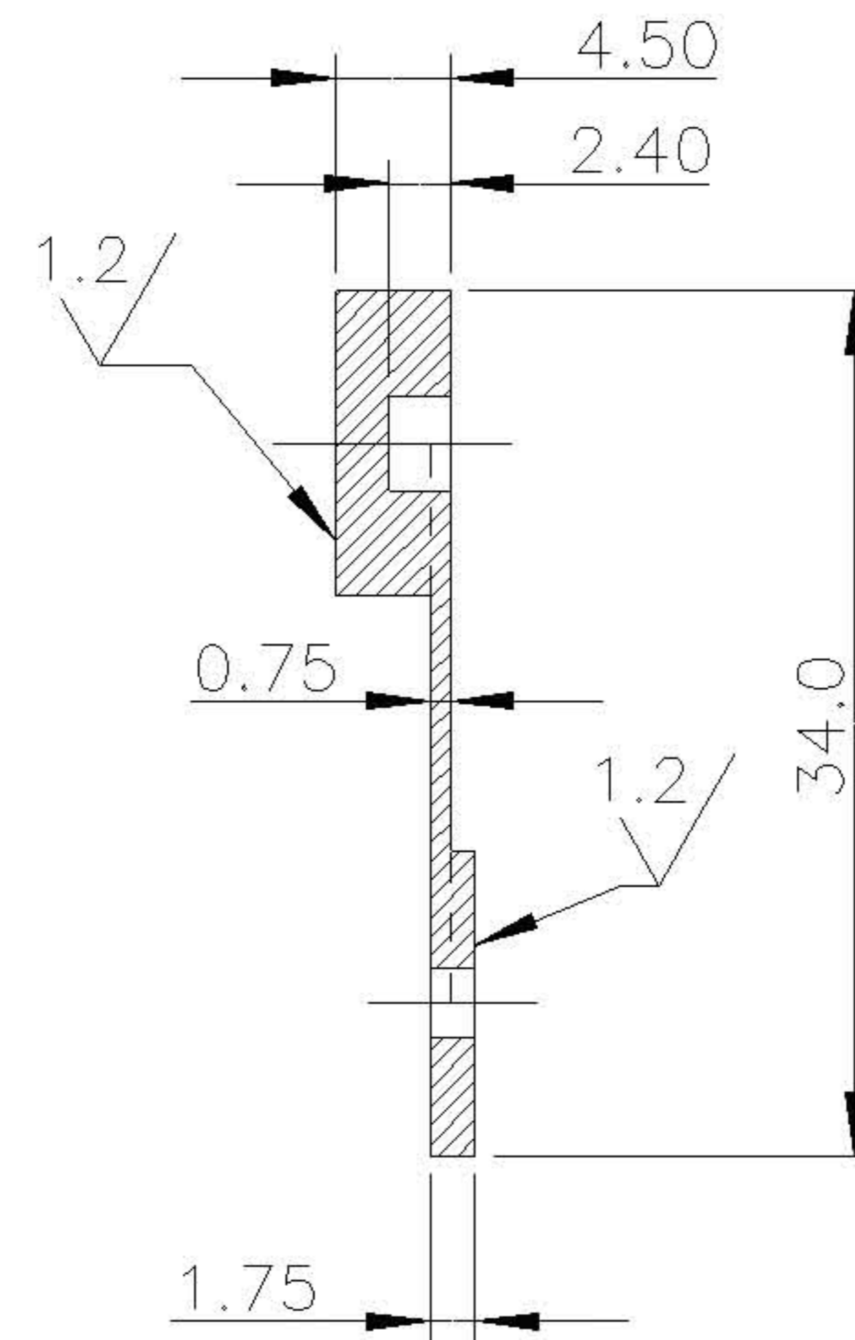
SECTION A-A
